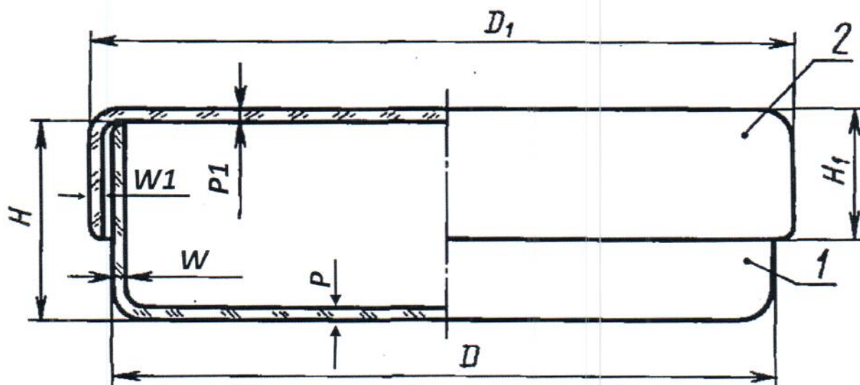
Рисунок 1 Чашка Петри в сборе
